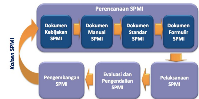
Gambar 2. Implementasi SPMI
