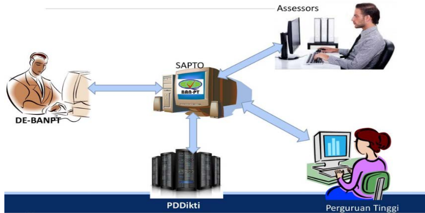
Gambar 14. Arsitektur SAPTO
